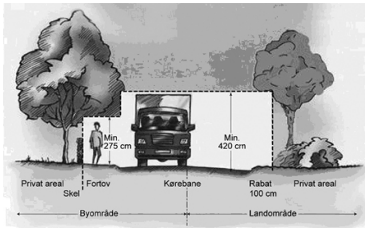
Principskitse for beskæring
